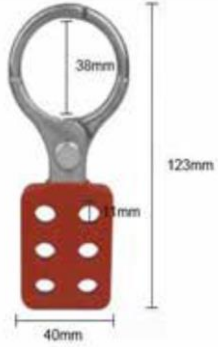
IS-K12 38mm Alüminyum Çene Çoklayıcı
