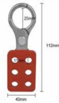
IS-K11 25mm Alüminyum Çene Çoklayıcı
